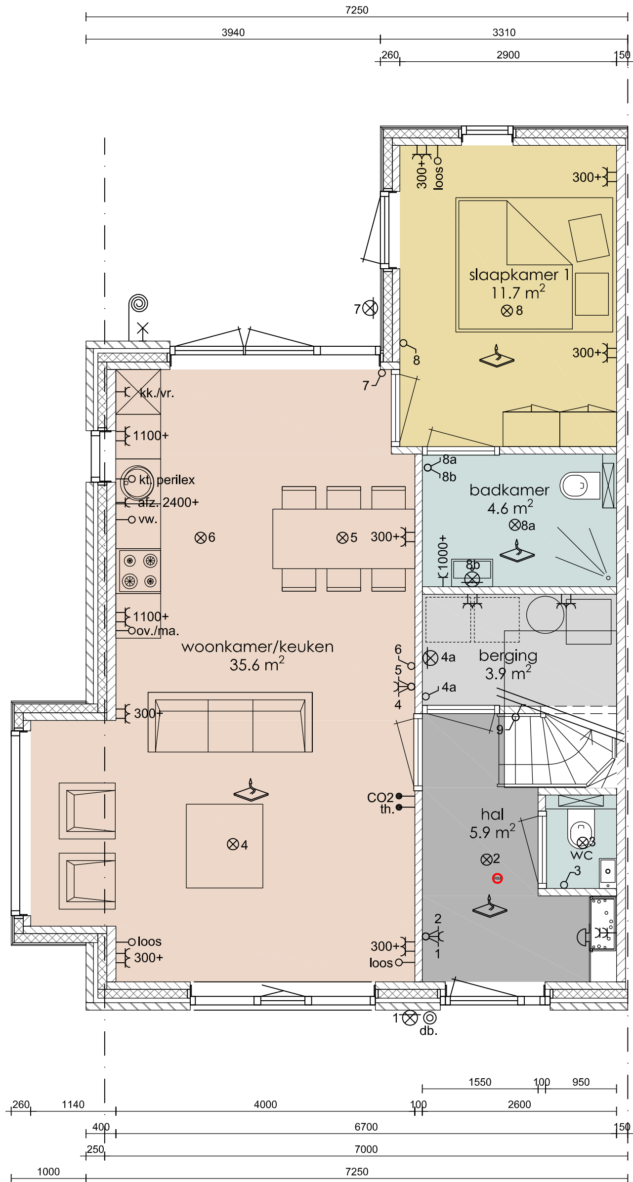
Eindwoning - begane grond levensloop slpk+badk variant incl. optie erker
