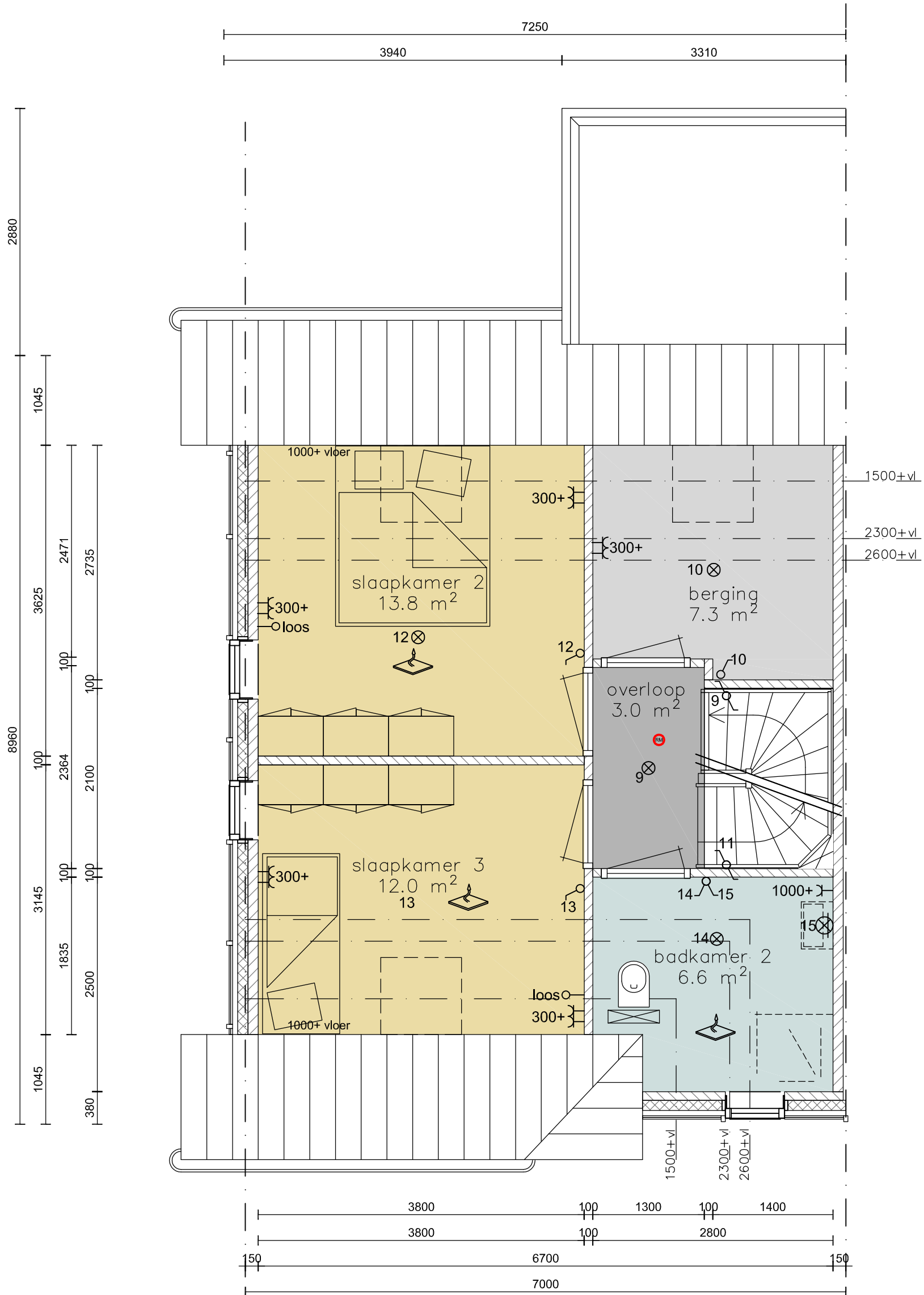
Eindwoning – verdieping levensloop badkamer variant
